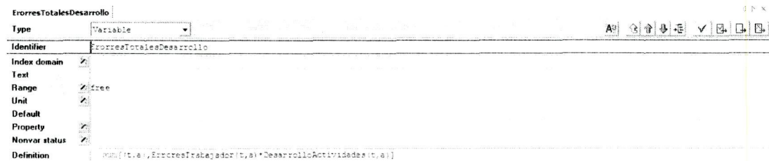
Figura 42. Variable que minimiza el número total de errores con base en el parámetro ErroresTrabajador(t,a).
