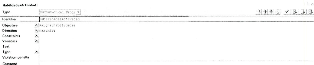
Figura 49. Función matemática para maximizar la asignación del nivel de habilidades en el desarrollo de las actividades a partir del parámetro NivelHabilidadesTrabajador(a,t) y de la variable AsignarHabilidades .
