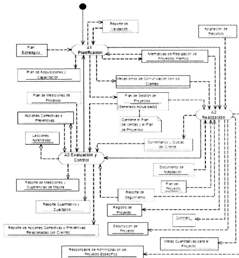
Figura 7. Diagrama de flujo de trabajo de la gestión de proceso.
