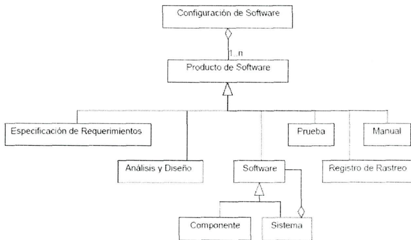
Figura 13. Ejemplo de clasificación de productos de software
