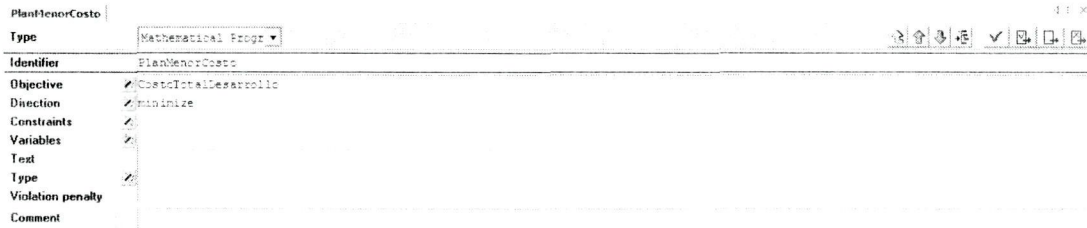
Figura 46. Función matemática para minimizar el costo total del proyecto a partir de los parámetros: TotalActividadesTrabajador(t,a) , TotalActividadesClase(a) y CostoUnitarioActividad(t,a) ; y a partir de las funciones: DesarrolloActividades(t,a) y CostoTotalDesarrollo .
