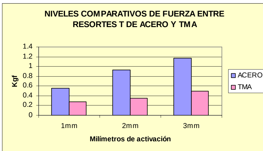
Grafico 4 Fuerza contra activación de resortes en T loop diseñados en alambre de SS y TMA calibre .016x.022 pulgadas
