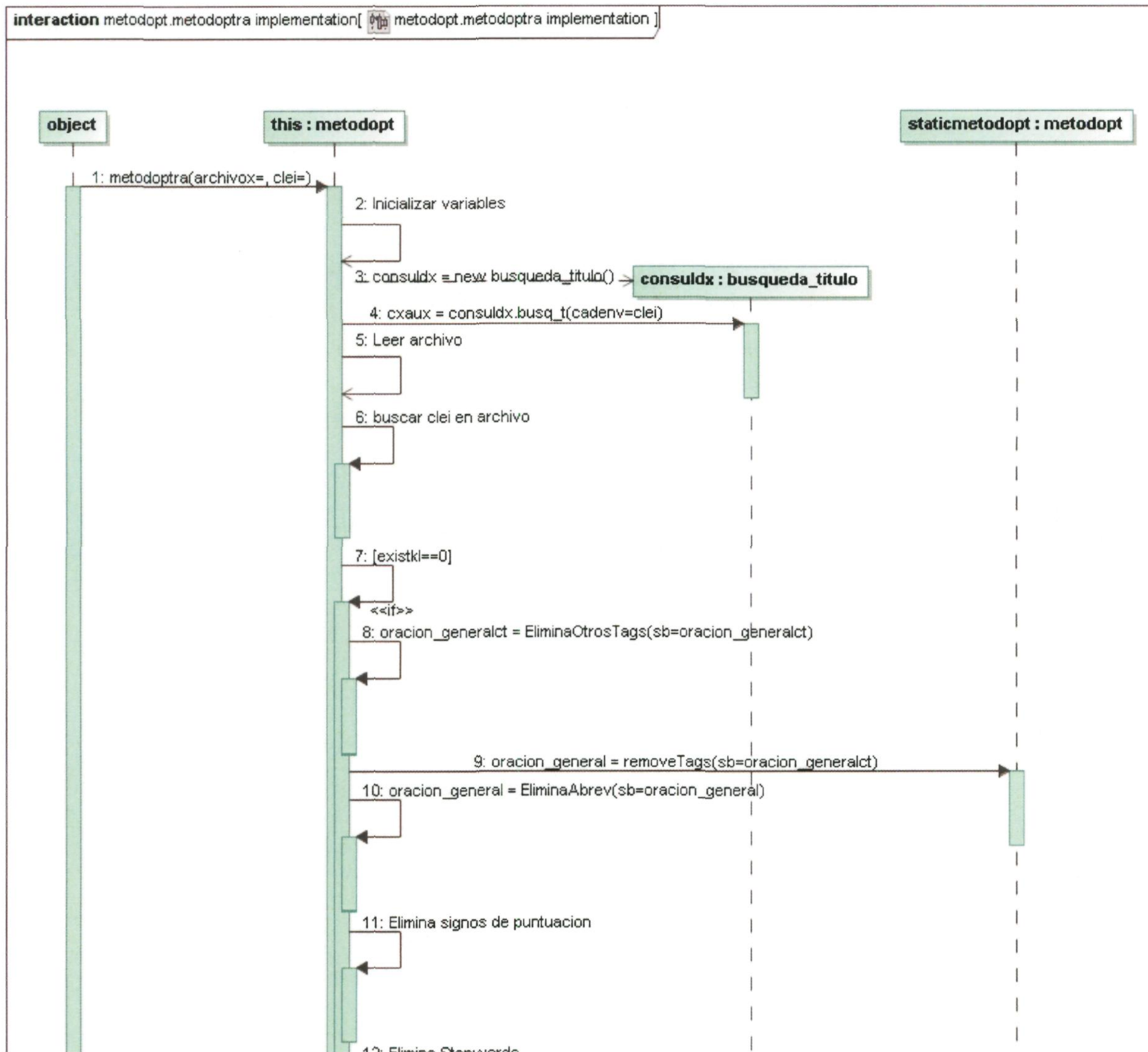
FIGURA 13. DIAGRAMA DE SECUENCIA PARA LA OPERACIÓN BUSCANDO DEL MÉTODO METODOPTRA
