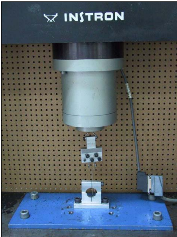
Fig. 12A Aparato universal de pruebas
