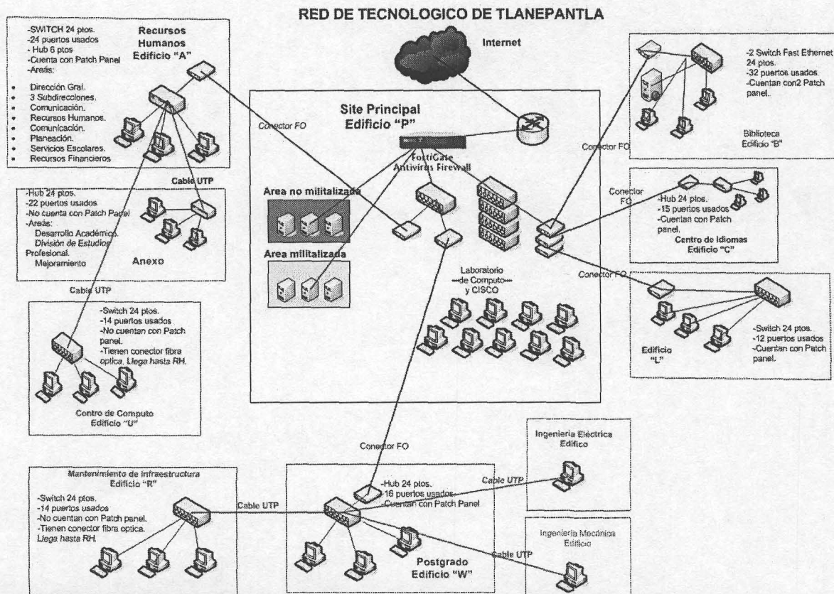
Figura 4. Diagrama de Red del ITTLA
