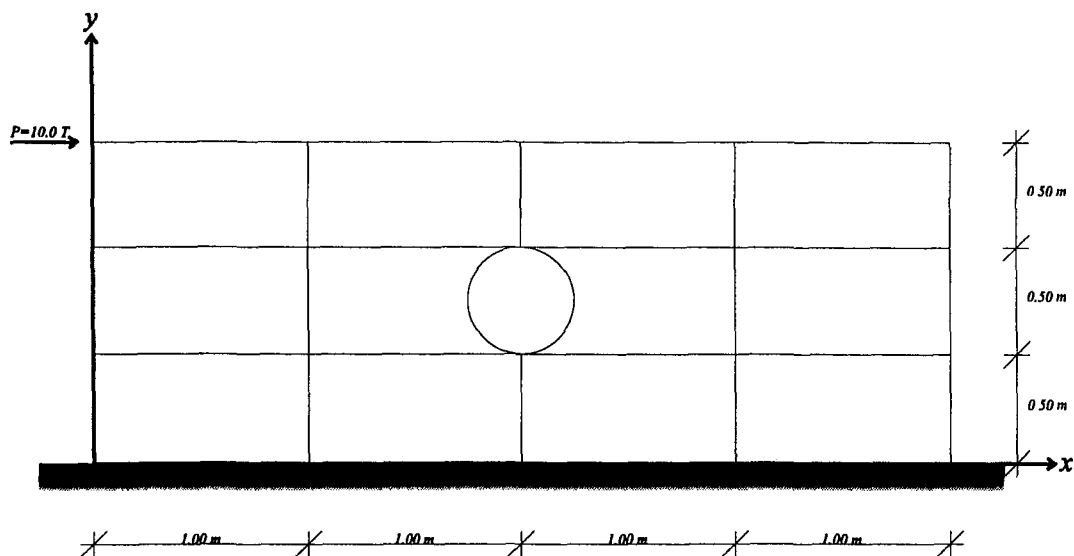
Fig 3.1 Diagrama del Muro a Analizar.
