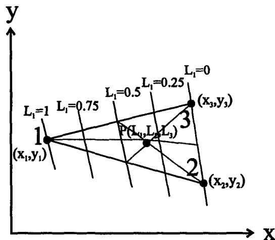
Fig. 2.4 Coordenadas de Área
