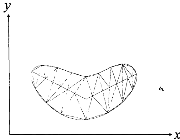
FIGURA 1.4 Región plana dividida en elementos finitos triangulares
