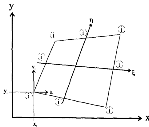
Fig 3.3 Coordenadas Globales del Elemento Finito tipo Cuadrilátero Cuadrático
