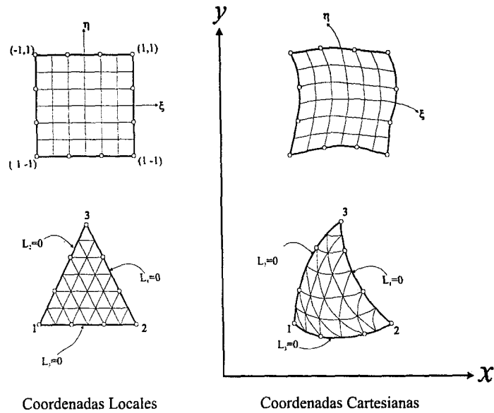
Fig 2.6 Mapeo de Elementos Bidimensionales
