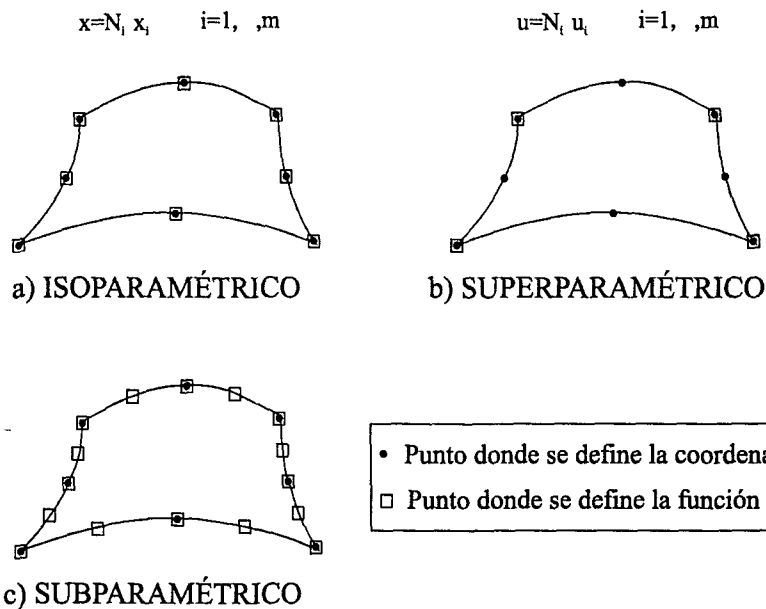
Fig. 2.7 Transformación de Coordenadas Mediante Funciones de Forma
