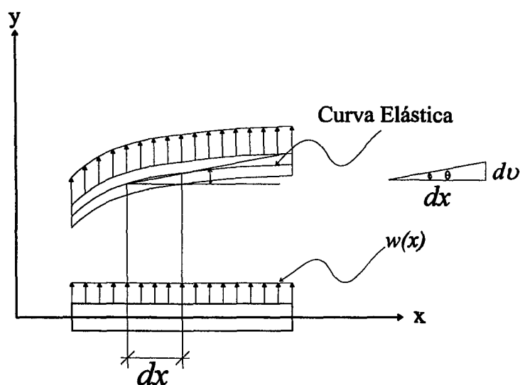
Fig. 2.1 Elemento diferencial de una viga cargada transversalmente
