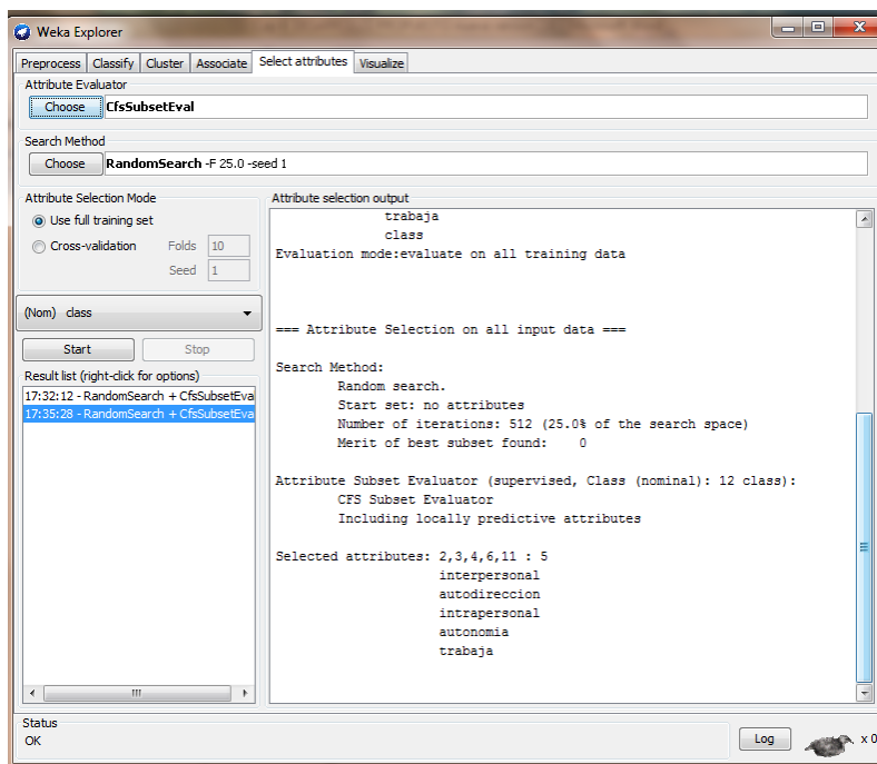
Figura 4.12 Ejecución del evaluador de atributos CfcssubsetEval
