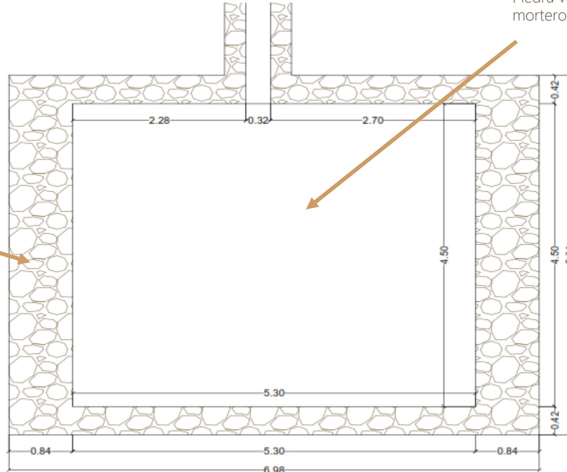
Planta
