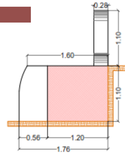
Alzado
