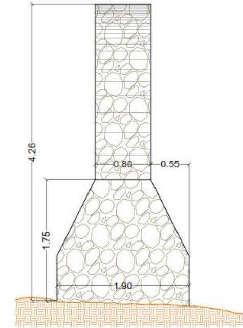
Corte del arco no. 2
