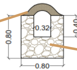
Detalle del caño que va hacia la arcada
