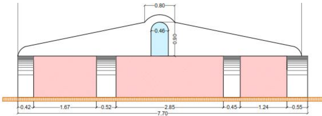
Fachada
