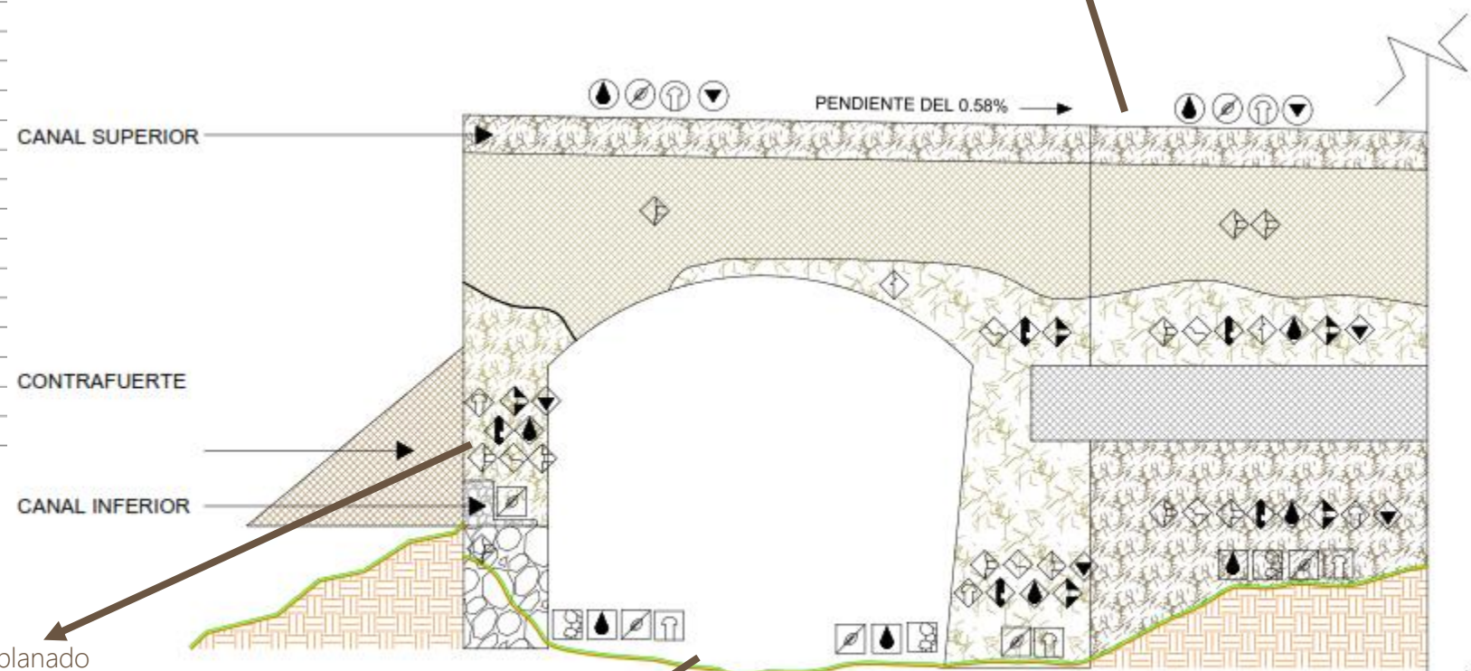
Vista posterior del arco no. 1 esc. 1:100
