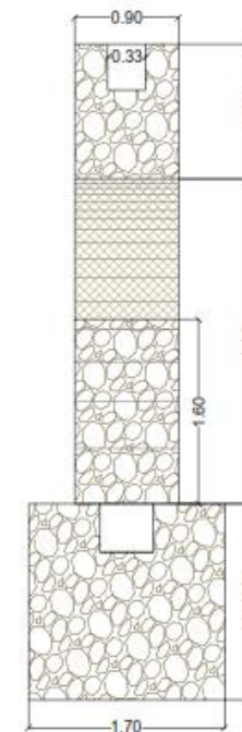
Vista interna del arco no. 2 esc. 1:100
