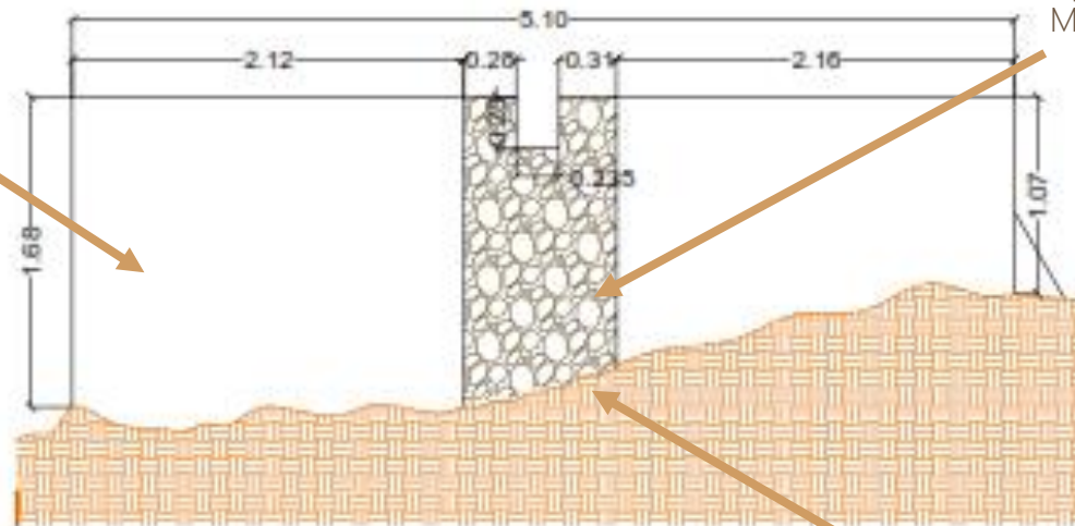
Vista Oriente
