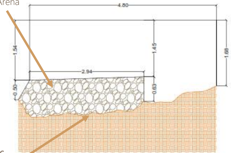
Vista Sur
