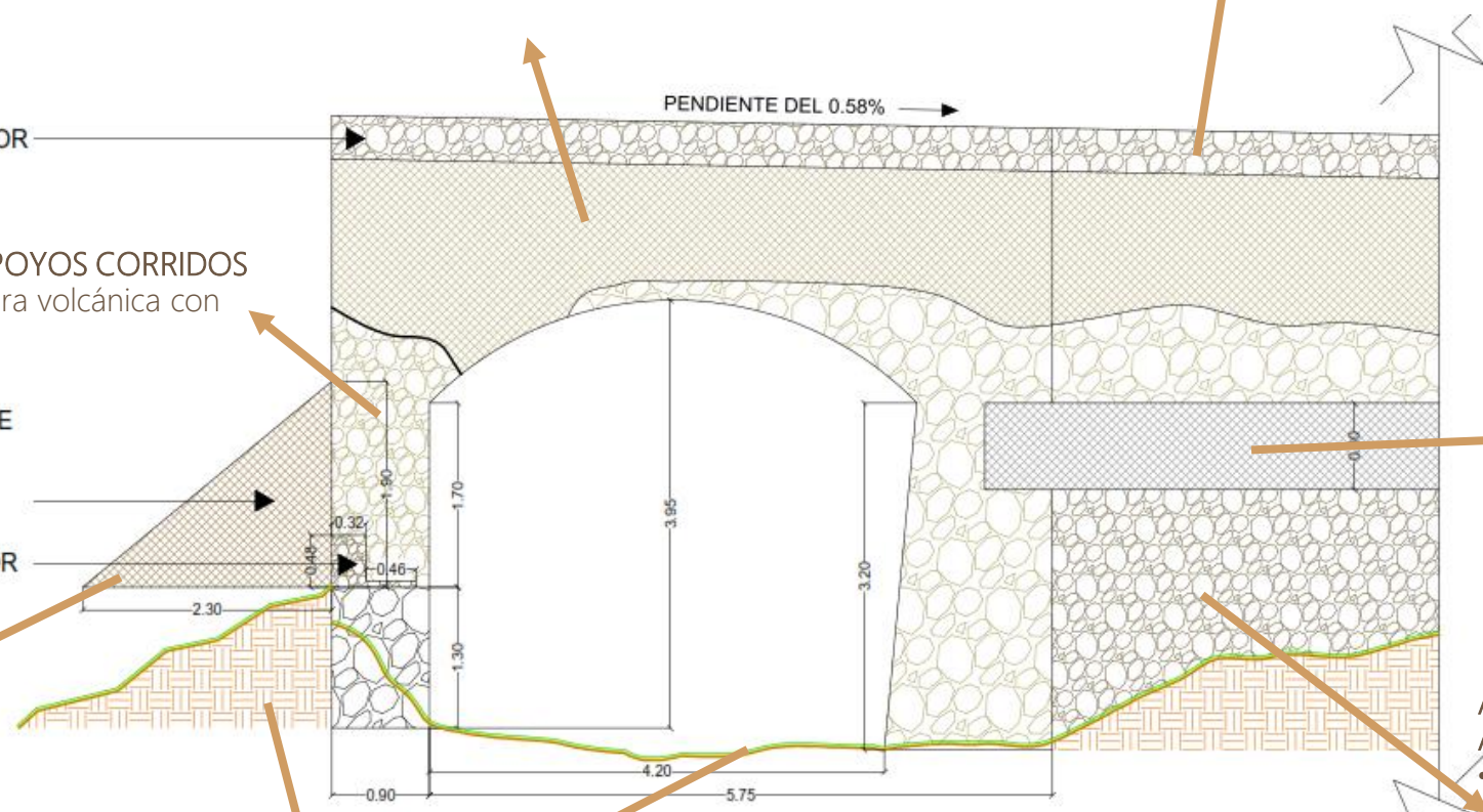
Vista posterior del arco no. 1 esc. 1:100
