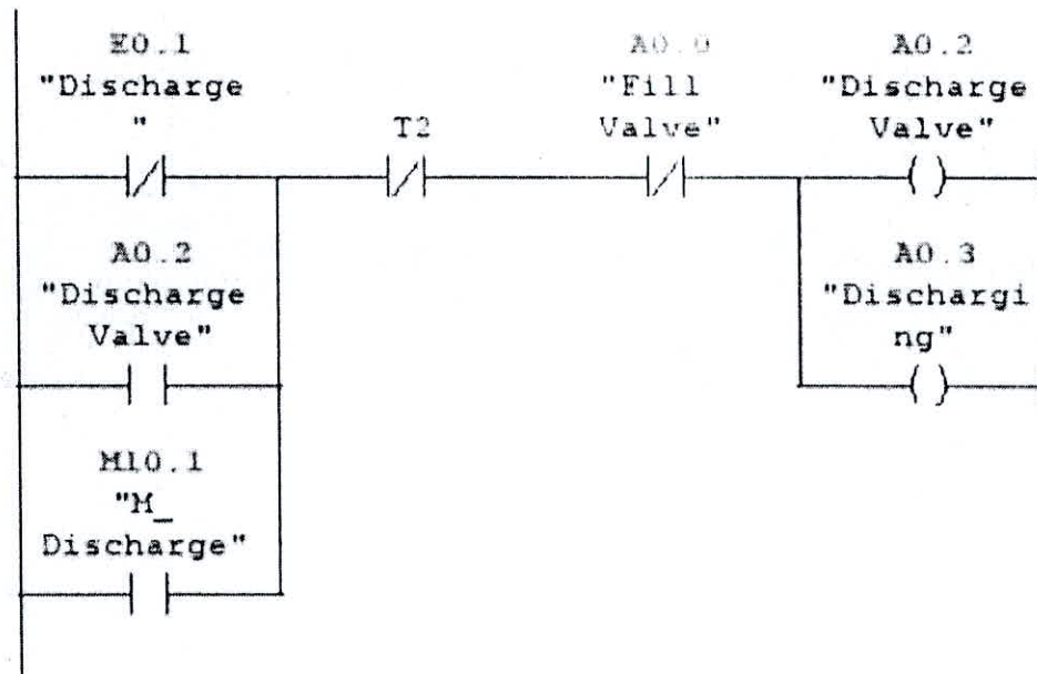
Ilustración 11: Una vez lleno utilizaremos nuestra válvula de descarga la cual será activada por un timer (T2) una vez lleno el tanque procederemos a vaciarlo activando nuestra válvula de vaciado conforme al tiempo determinado con nuestro timer
