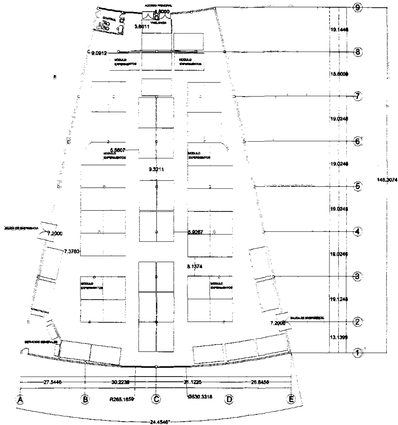
PABELLON DEL HOMBRE PLANTA (tipo)
