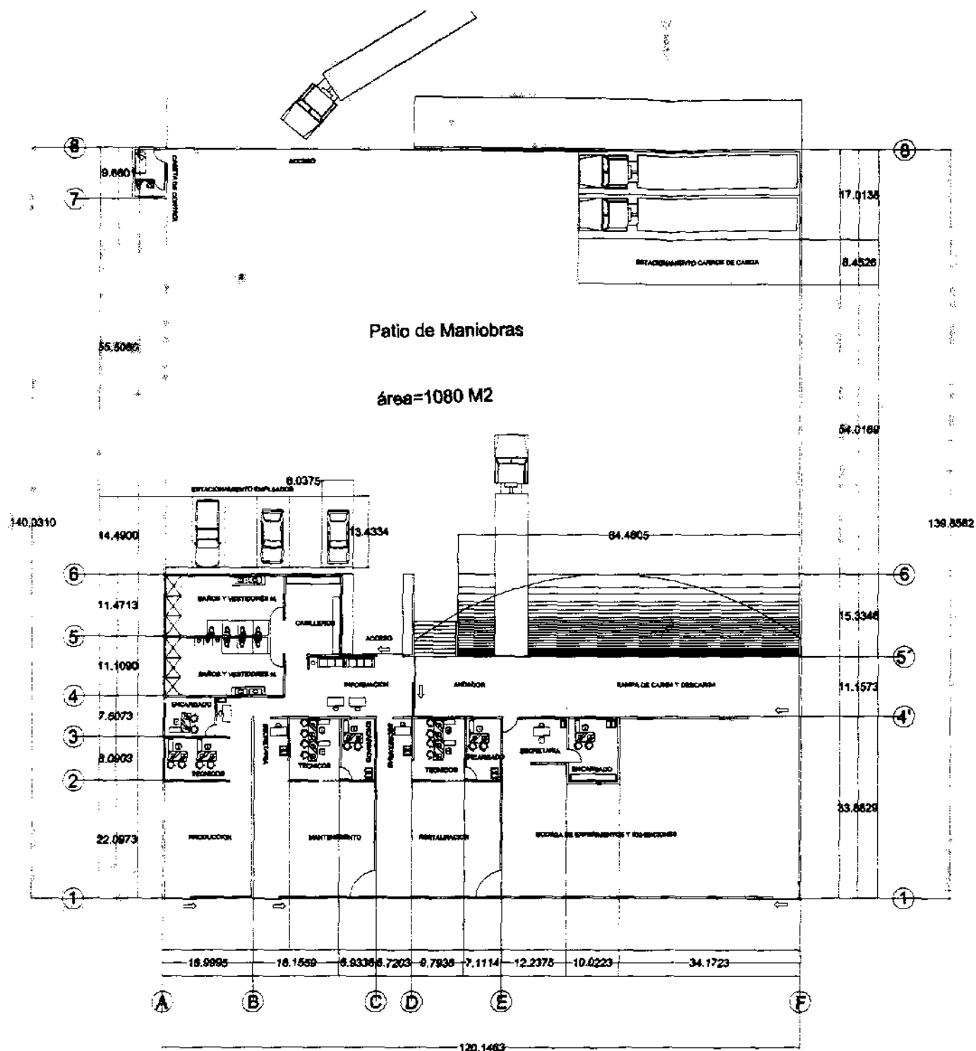
PLANTA ARQUITECTONICA BODEGAS Y TALLERES
