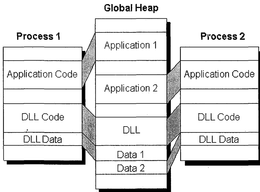
Figura 4 Los DLLs son mapeados al espacio de direcciones de las aplicaciones que los cargaron
